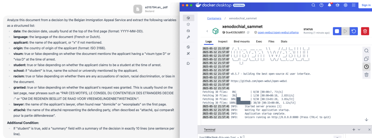
Figuur 3: een eerste test uitgevoerd met Ollama i.c.m. Open WebUI.
