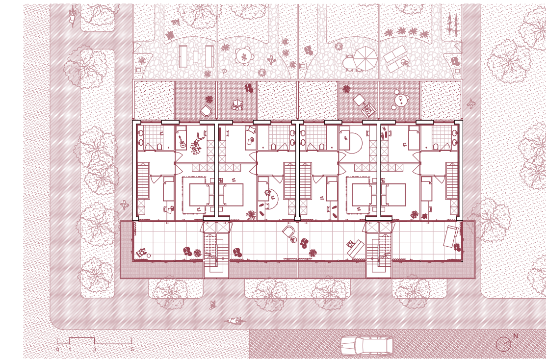
Figuur 4.54 Niveau +1
