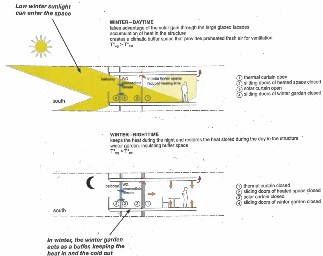
Technische werking van de wintertuin in de winter
