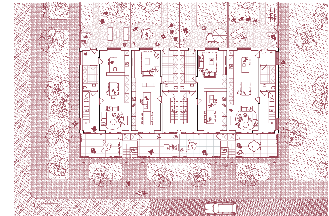
Figuur 4.53 Niveau 0
