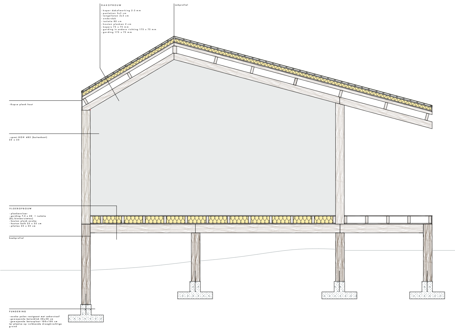
Figuur 2.32 Detailsnede
