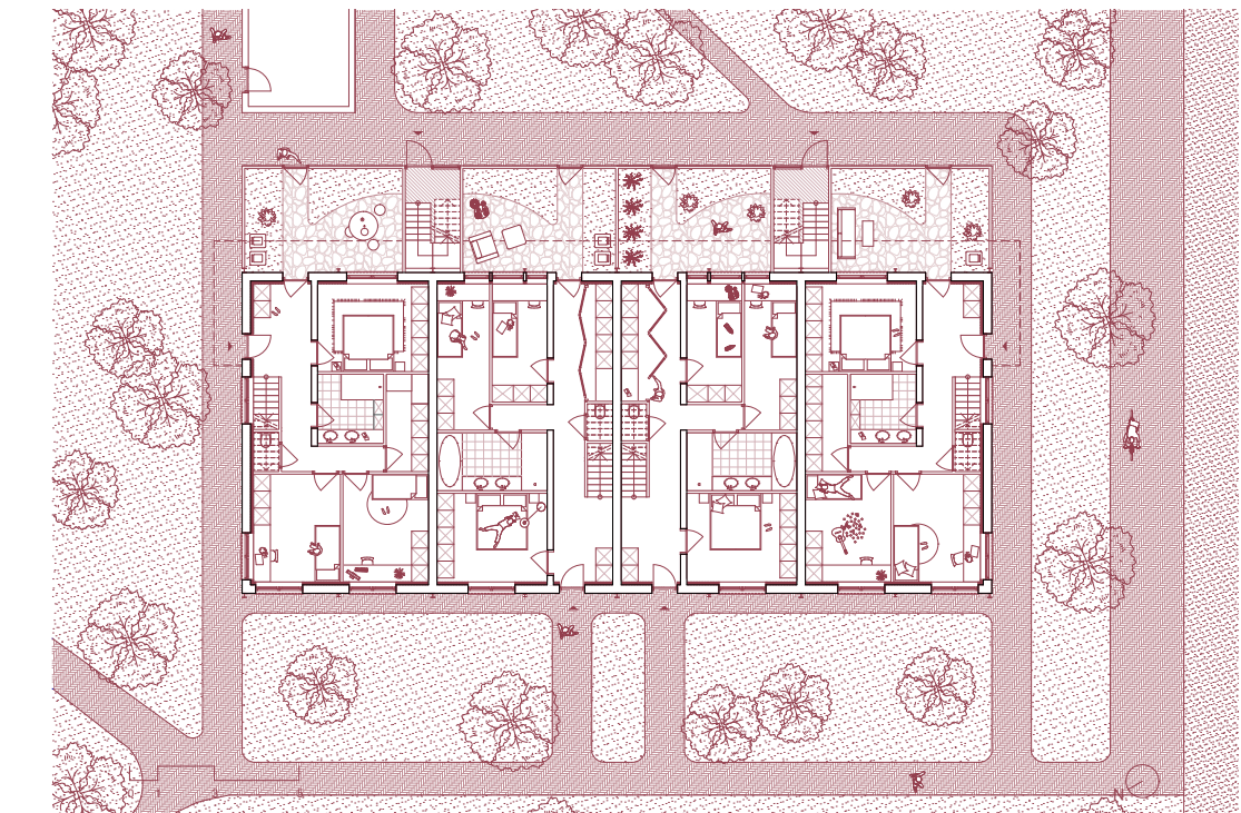
Figuur 4.58 Niveau 0
