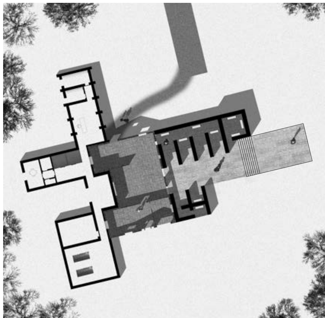
Figuur 1.53 Grondplan dierencrematorium
