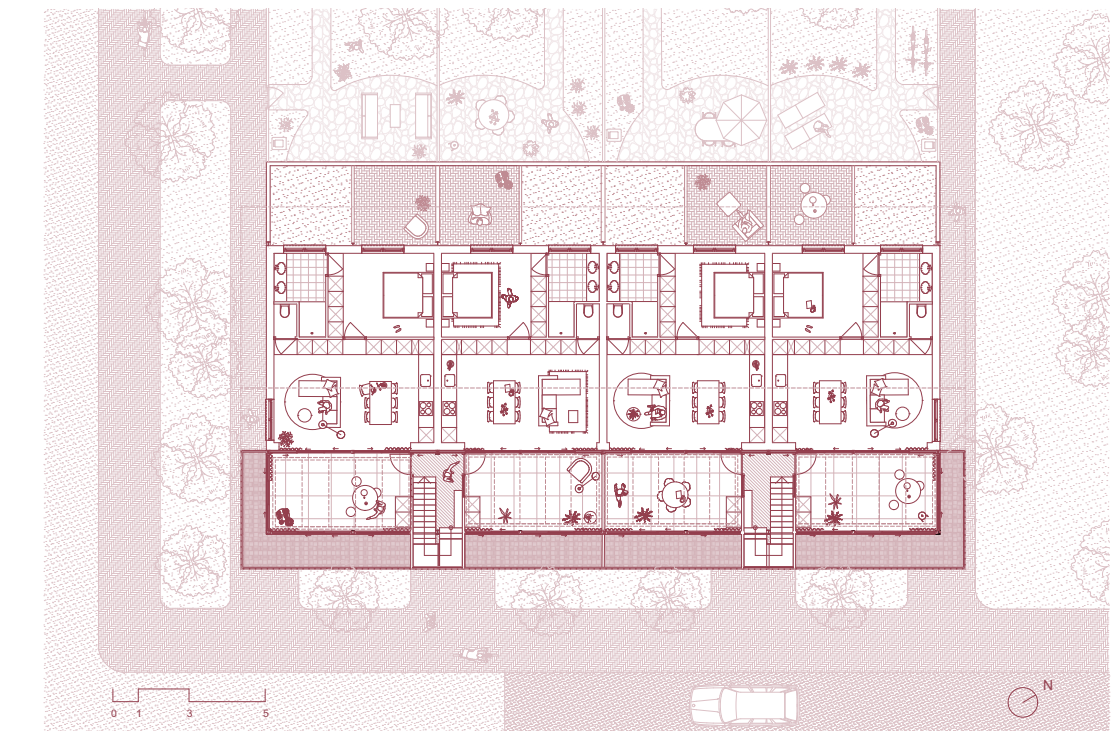
Figuur 4.55 Niveau +2
