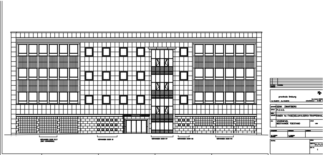
Figuur 3.28 Oude geveltekening PLOT-hoofdgebouw (voorgevel)
