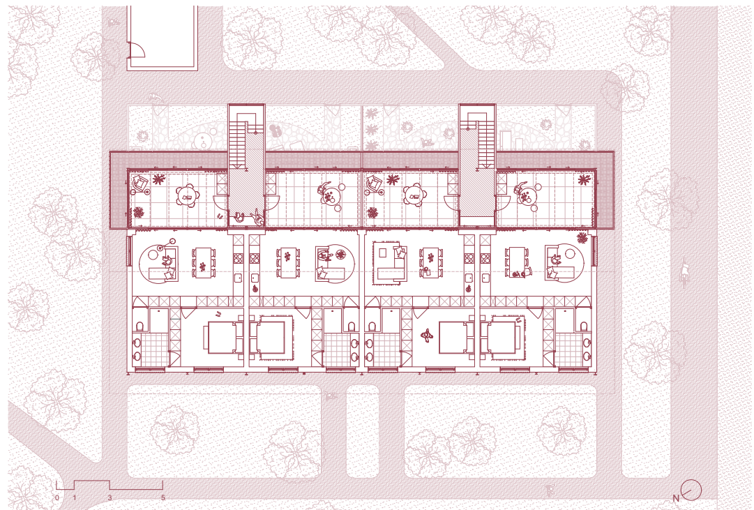
Figuur 4.60 Niveau +2
