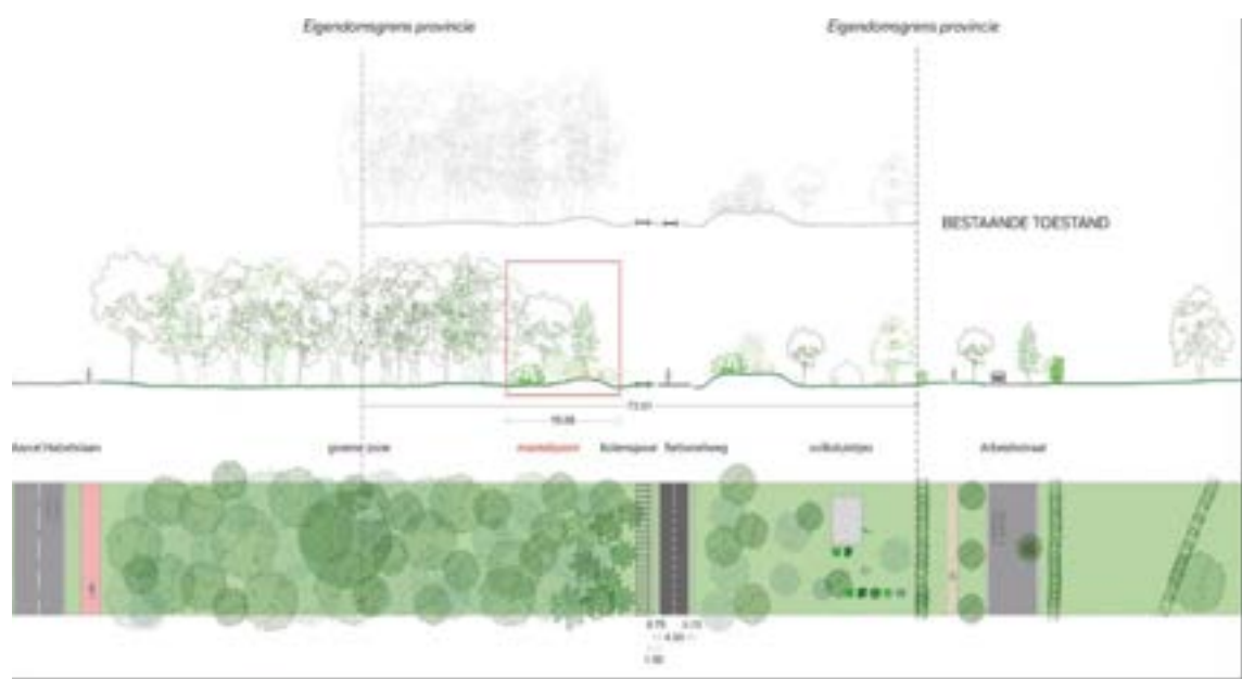
Figuur 3.25 Opbouw en dwarsdoorsnede fietssnelweg
