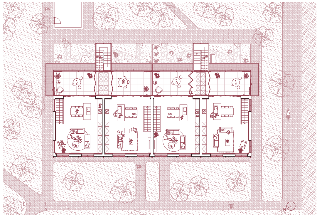
Figuur 4.59 Niveau +1
