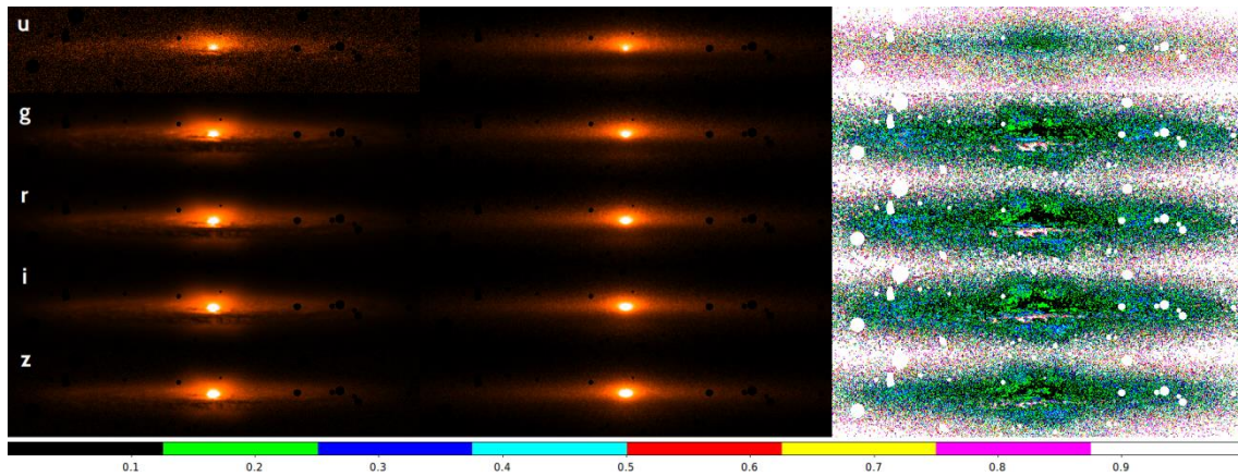
Figuur 5: Observaties (links), modellen (midden) en residuele beeld (rechts) van NGC 5746 in 5 verschillende golflengtebanden.
