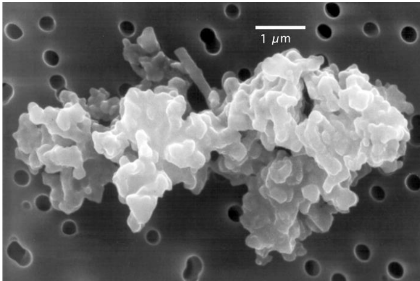
Figuur 1: Voorbeeld van een interstellair stofdeeltje.
