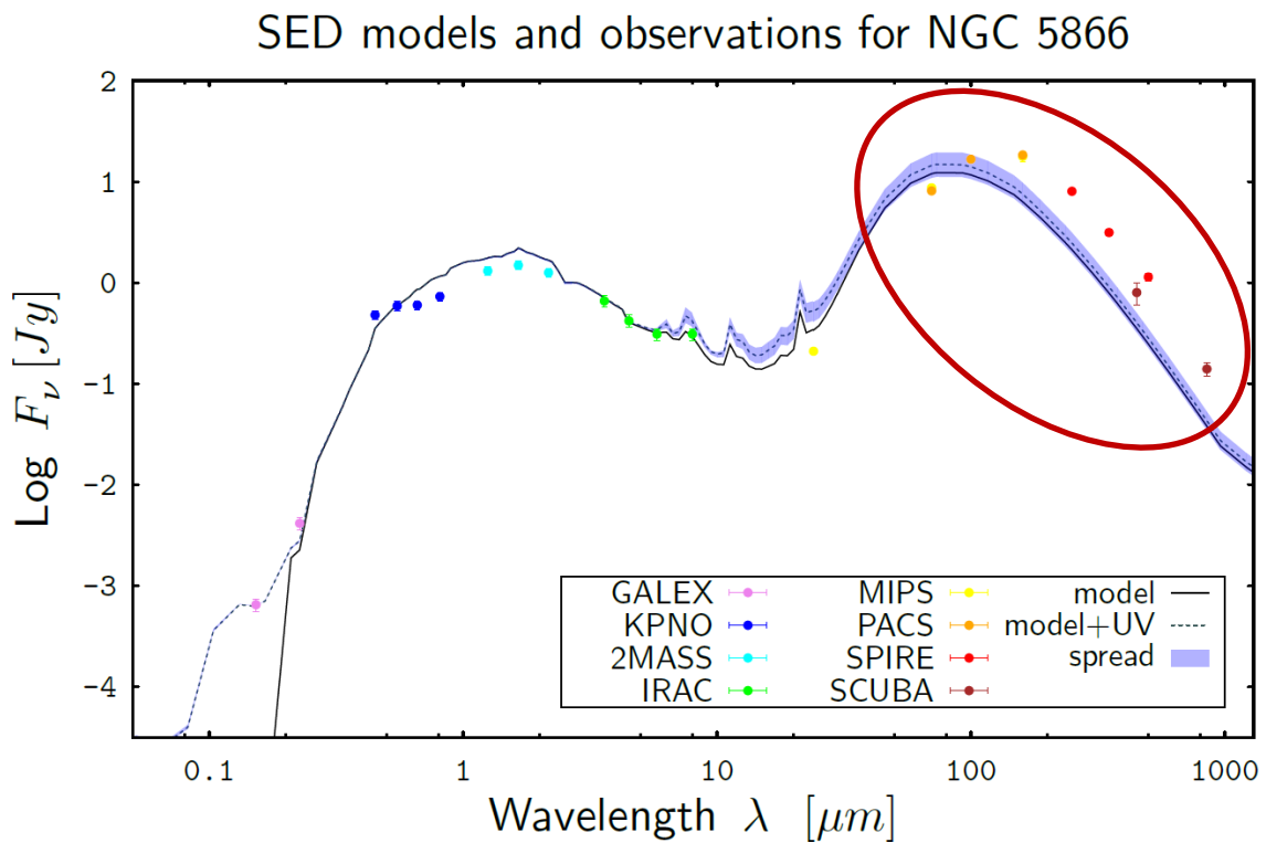
Figuur 6: Vergelijking tussen de voorspelde (lijnen) en de waargenomen (bolletjes) emissie van NGC 5866. Het is duidelijk dat de voorspelling de waargenomen emissie onderschat bij relatieve grote golflengtes (rode ovaal).
