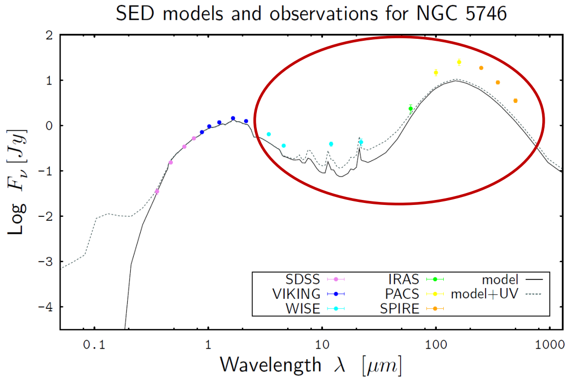
Figuur 7: Vergelijking tussen de voorspelde (lijnen) en de waargenomen (bolletjes) emissie van NGC 5746. Het is duidelijk dat de voorspelling de waargenomen emissie onderschat bij relatieve grote golflengtes (rode ovaal).
