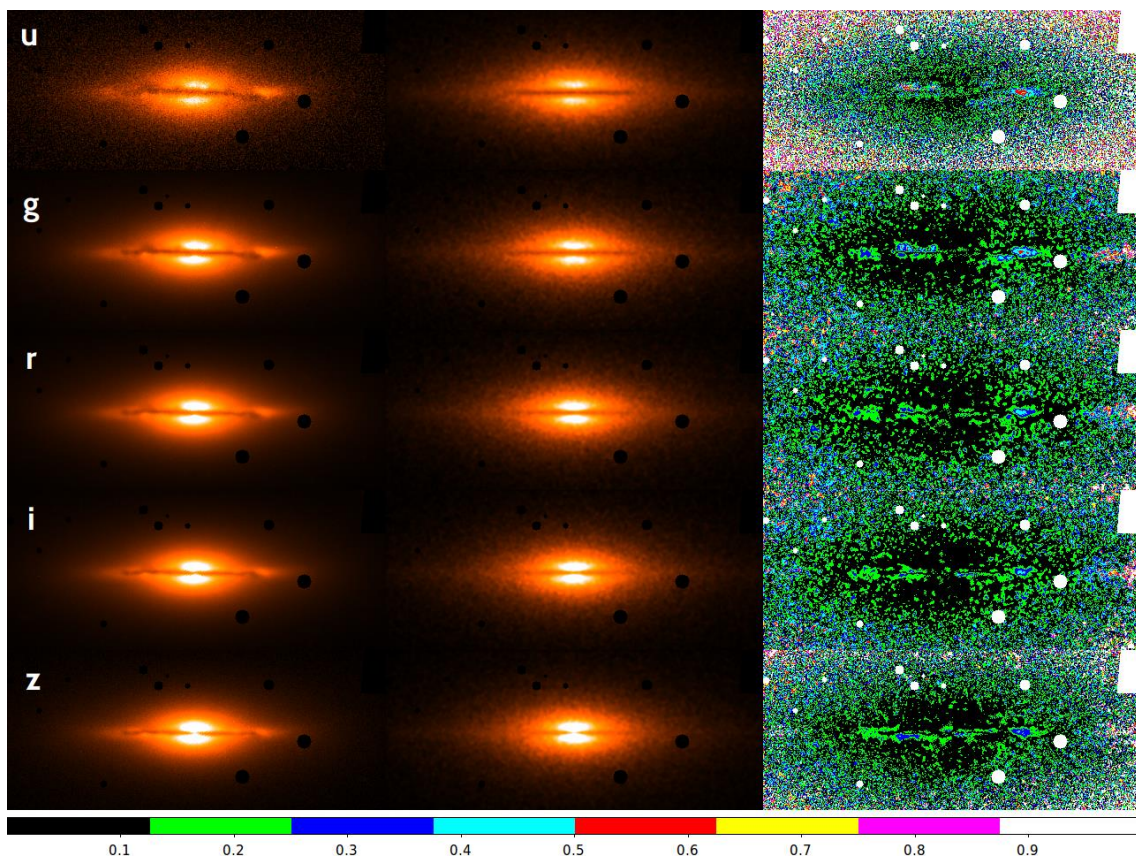
Figuur 4: Observaties (links), modellen (midden) en residuele beelden (rechts) van NGC 5866 in 5 verschillende golflengtebanden.
