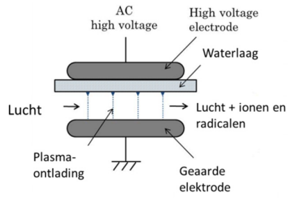
Figuur 1: Schematische voorstelling van plasma ontlading
