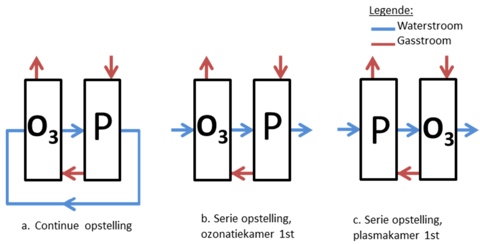
Figuur 2: Volledige reactor met verschillende configuraties
