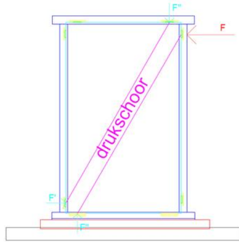
Figuur 1: constructieve diagonaal in het glas
