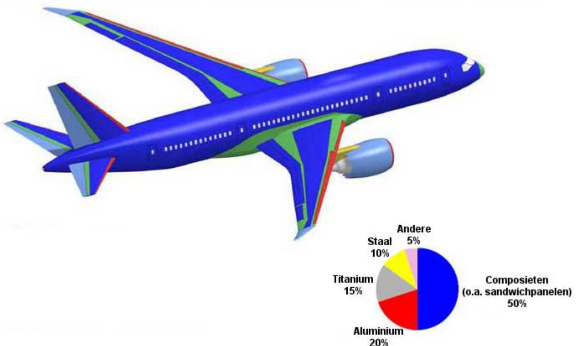
Figuur 2: het vliegtuig van de (nabije) toekomst zal grotendeels bestaan uit lichtgewicht composieten zoals sandwichpanelen. Deze schets toont het materiaalgebruik in de Boeing 787, een nieuw vliegtuig dat gedeeltelijk werd opgebouwd uit composieten. (Oorspronkelijke afbeelding afkomstig van Boeing, http://www.boeing.com )
