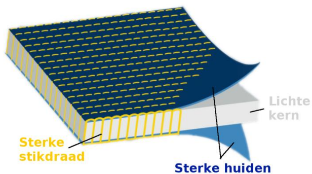
Figuur 1: voorstelling van een gestikt sandwichpaneel waarbij twee sterke huiden aan een kern worden gestikt (links) en de oplegger bestaande uit sandwichpanelen gebouwd door Acrosoma (rechts). (Oorspronkelijke afbeeldingen afkomstig van Acrosoma, http://www.acrosoma.com )
