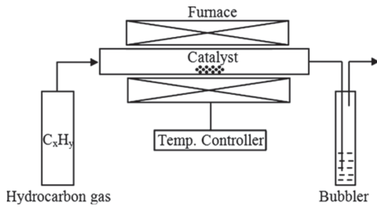
Figuur 4: Schematische voorstelling van een eenvoudig CVD toestel.
