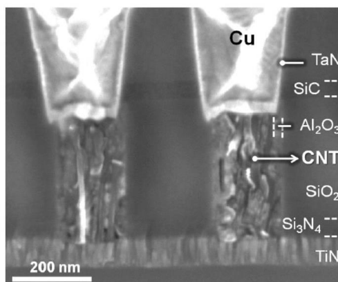
Figuur 7: Elektronenmicroscop afbeelding van koolstof nanobuizen geïntegreerd als interconnects.
