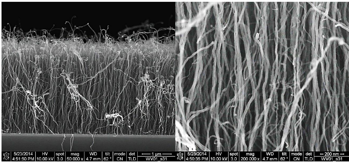
Figuur 6: Elektronenmicroscop afbeelding van een tapijt aan koolstof nanobuizen. Een overzicht (links). Close-up (rechts).
