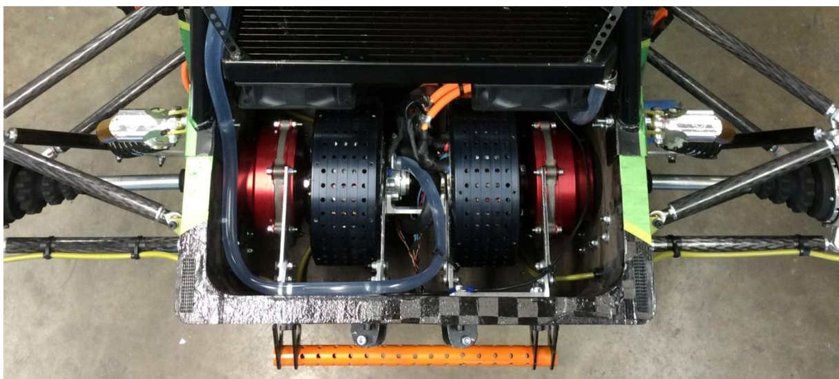
Figuur 4. De ontworpen transmissies met motoren vanachter in de wagen.
