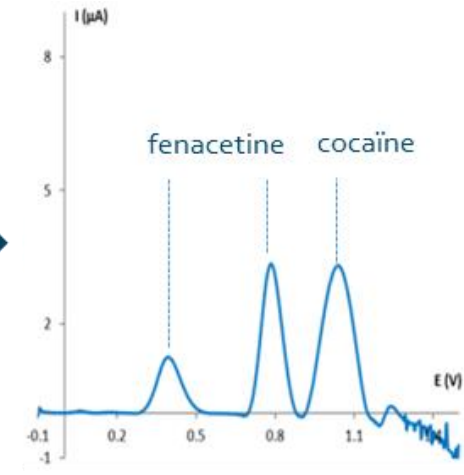
Elektrochemische handtekening van het verdachte poeder met 73% cocaïne en 17% fenacetine.
