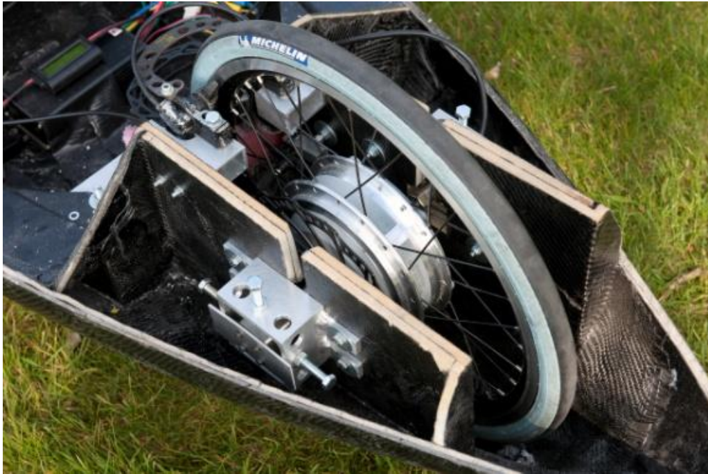
Figuur 2: Bafang hub motor bevestigd op een 3D regelbare ophanging
