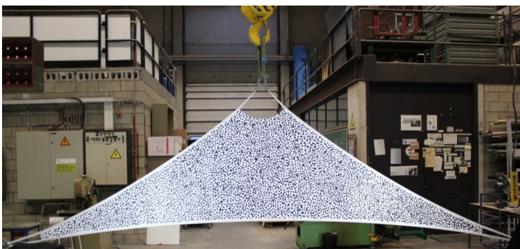
De testopstelling: een driehoekig membraan, opgehangen aan de hoekpunten en belast in de top.
