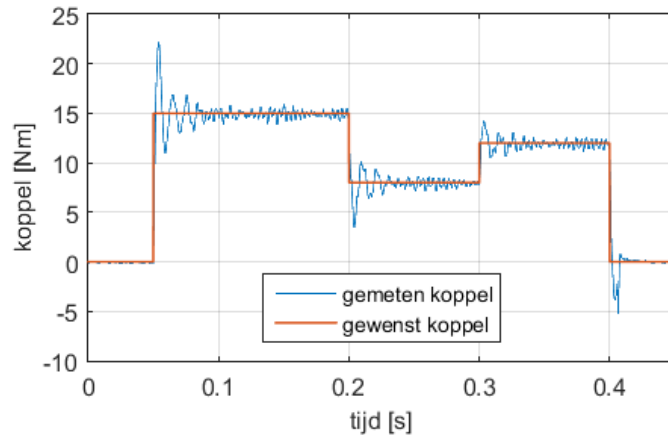
Figuur 1: PI-regelaar
