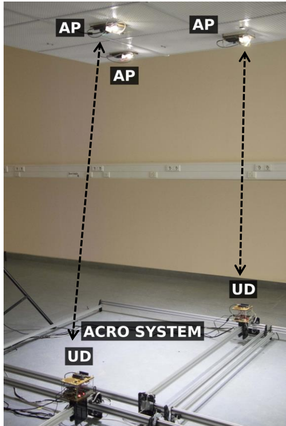
Figuur 3: experimentele opstelling voor LightTour. AP = LED-lamp, UD = gebruikerstoestel, het ACRO systeem verplaatst de gebruikerstoestellen op voorgeprogrammeerde routes.
